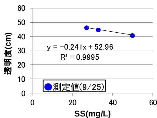
図-2 SS 濃度と透明度との関係
