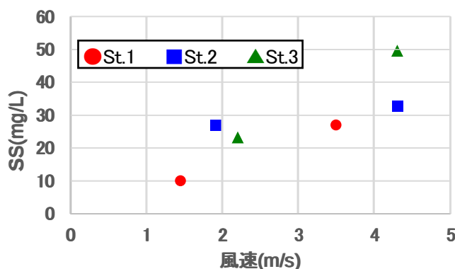
図-1 風速と SS 濃度との関係
